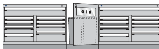
2 coffres à outils - Panneau et contenants pour rebuts et récupération
