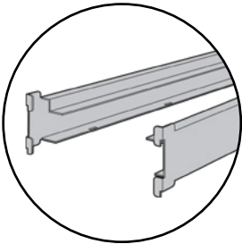
La prise par « griffes » des poutrelles aux montants assure une structure rigide assemblée en quelques instants.
